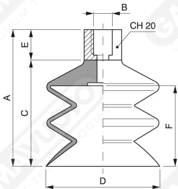
Art. SF 43 02 - SF 60 02 - SF 85 01
